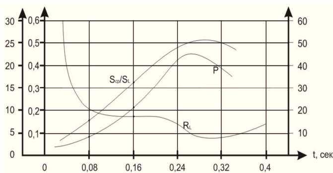
Рис. 2. Характер изменения прочности (P) и электросопротивления (R k ) контакта, отношения площади сварного соединения (S св ) к общей площади контакта S к от времени (t) для контактных пар Al-Al при УЗ-микросварке
