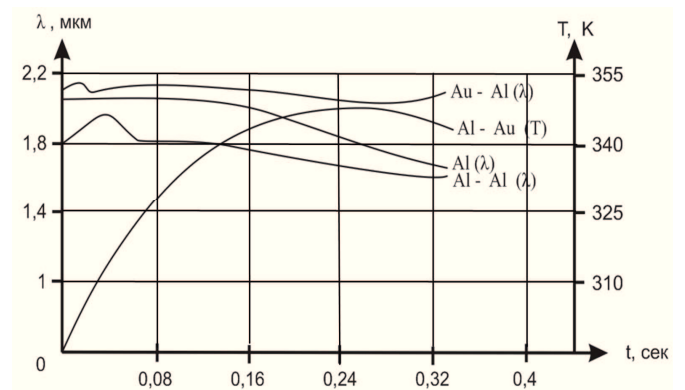
Рис. 3. Характер изменения температуры T и амплитуды колебаний (λ) для контактных пар при ультразвуковой сварке
